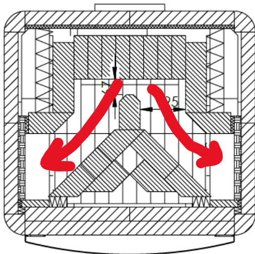
SECTION 9-9 SCALE 1 : 17
